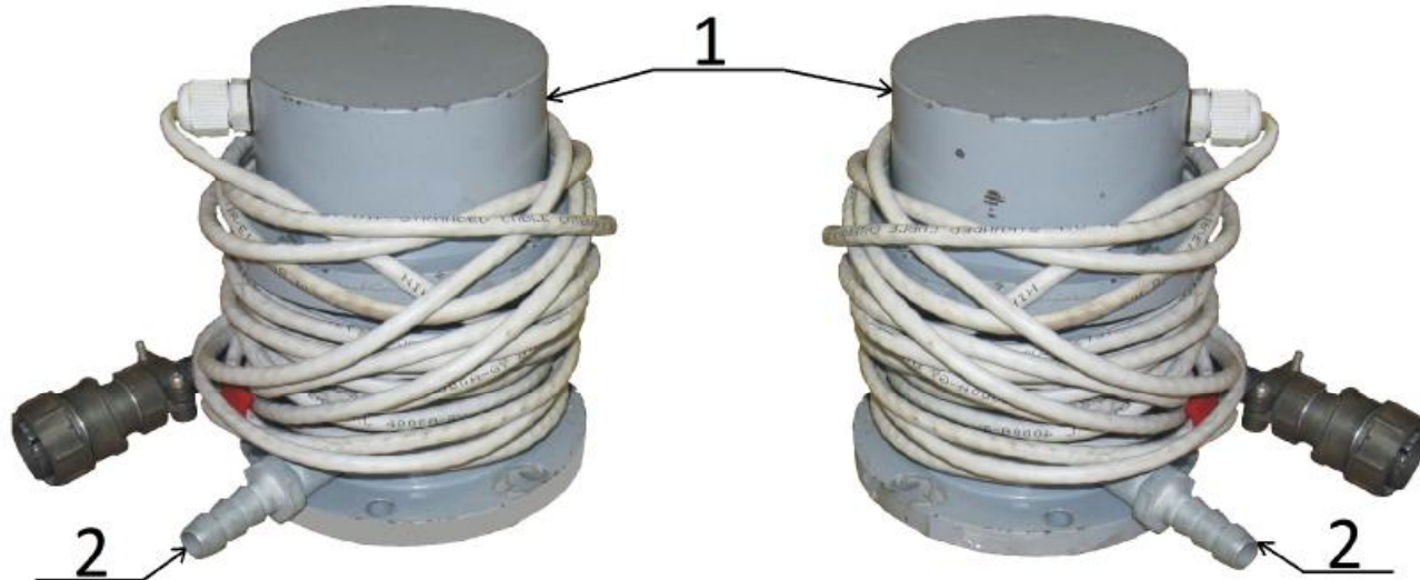
Рисунок 2 – внешний вид датчиков измерительных 1 – датчик измерительный; 2 – штуцер подачи сжатого воздуха.
